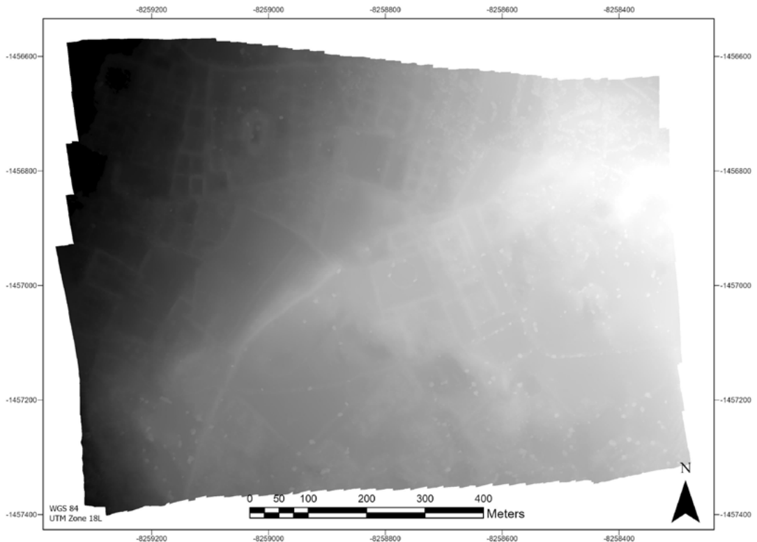
Figura 14. Detalle del modelo de elevación digital (DEM) ortorectificado y georreferenciado del Paso 4, que revela probables alineaciones arquitectónicas ocultas por la cubierta vegetal.
