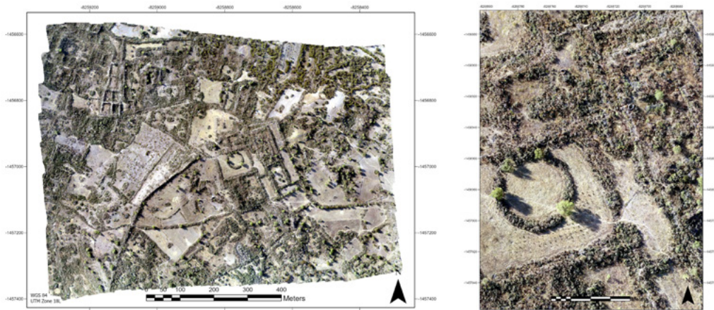
Figura 13. Imágenes ortorectificadas y georreferenciadas del sector Capillapata, mostrando el Paso 4 (izquierda) y detalles del Paso 4 (derecha).
